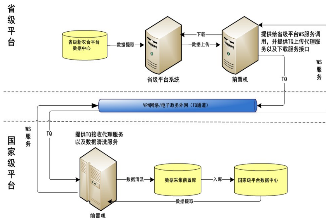
图-1 省级平台数据交换流程图
